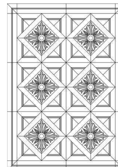
Модуль Фальер и бордюр Перье
