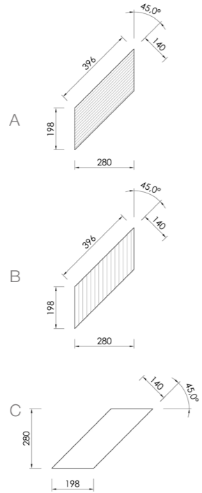
Конструкция деревянной плитки из коллекции Александра Эрмана
